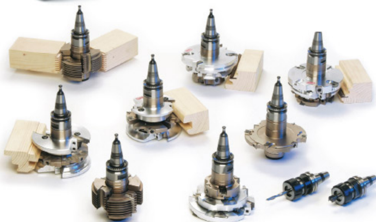
Jeux d'outils pour usinage sur CN
